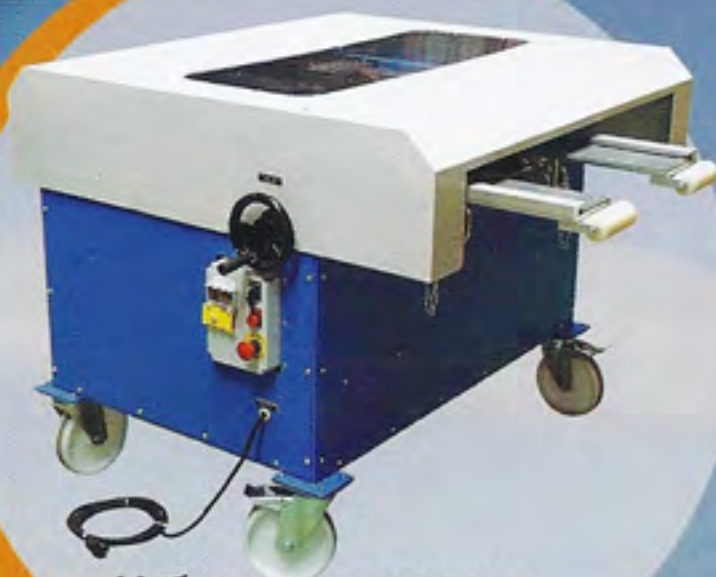
Мобильные кровельные станки
